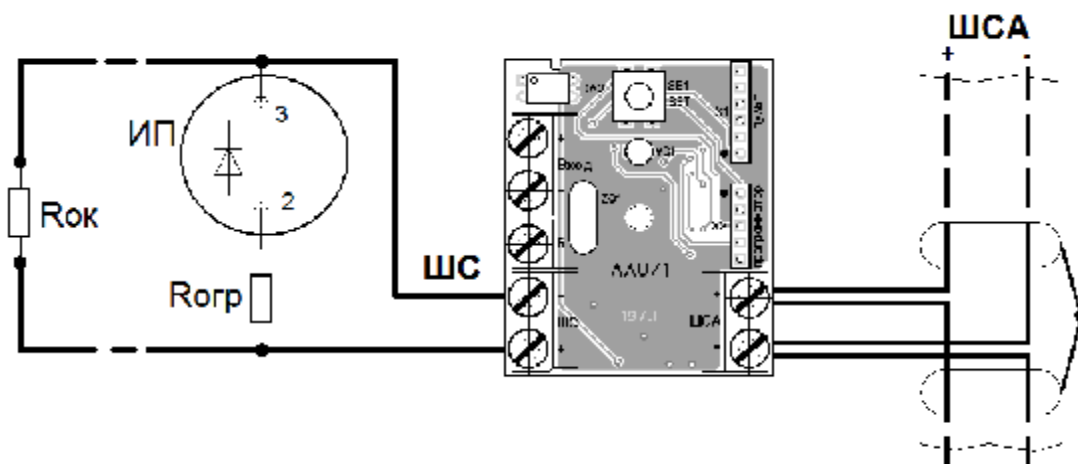
Рисунок П4 - Схема подключения извещателей (активных, работающих на увеличение тока в ШС и имеющих падение напряжения от 5 В до 8 В в режиме "Тревога")
