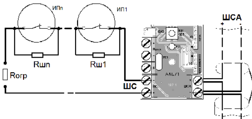
Рисунок П6 - Схема подключения извещателей, не потребляющих ток от ШС, выключателей и кнопок управления, работающих на уменьшение тока в ШС и имеющих НЗ контакт.
