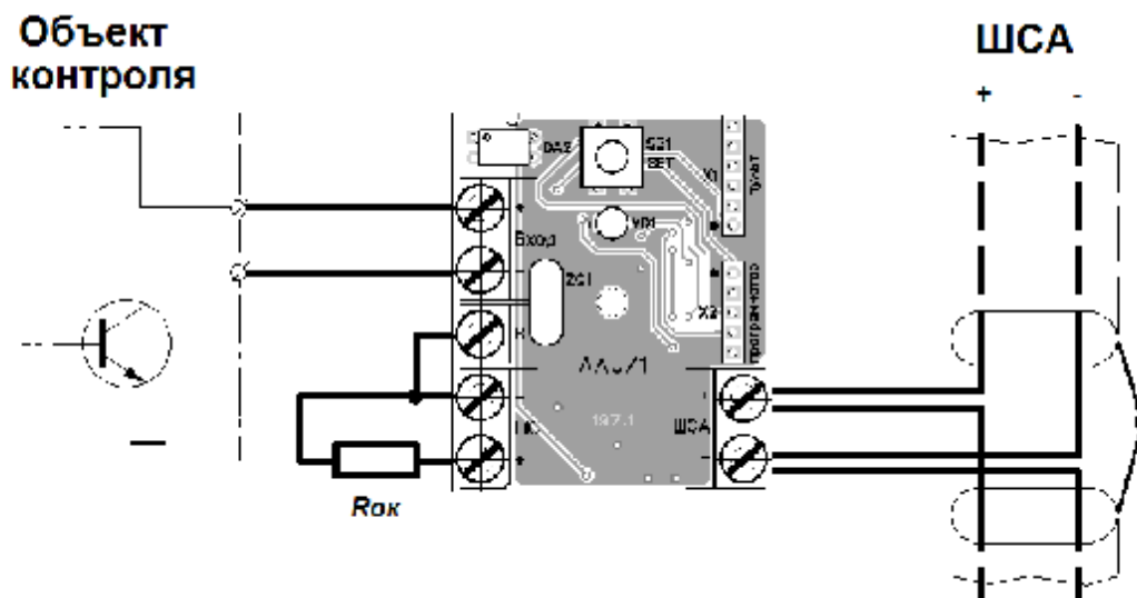
Рисунок П7 - Схема подключения ААУ к объекту контроля (сенсору) и ШСА
