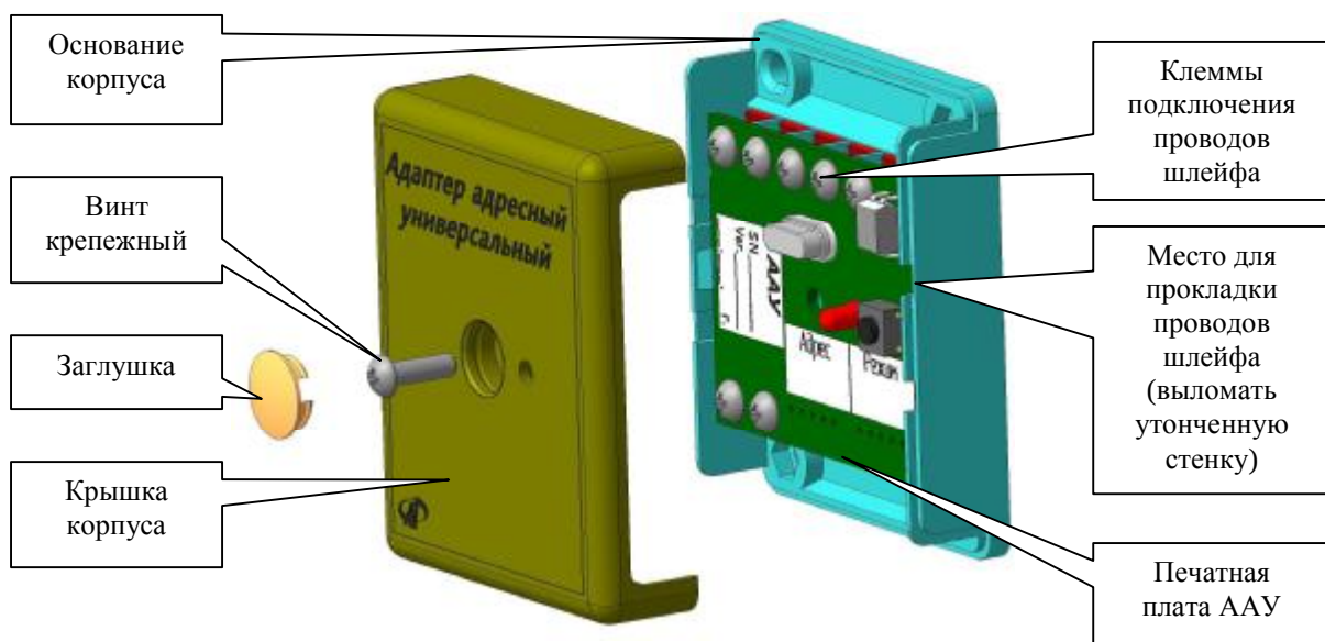
Рисунок П2 - Общий вид и конструкция ААУ
