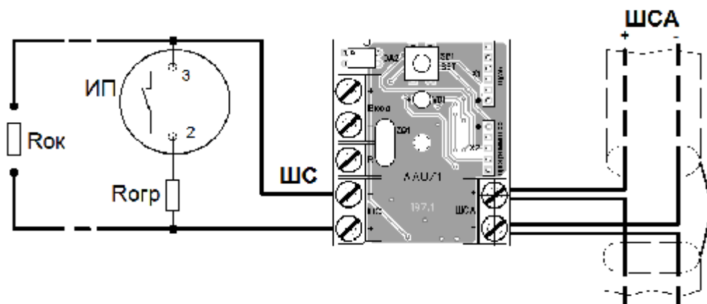
Рисунок П5 - Схема подключения извещателей, не потребляющих ток от ШС, выключателей и кнопок управления, работающих на увеличение тока в ШС и имеющих НР контакт.
