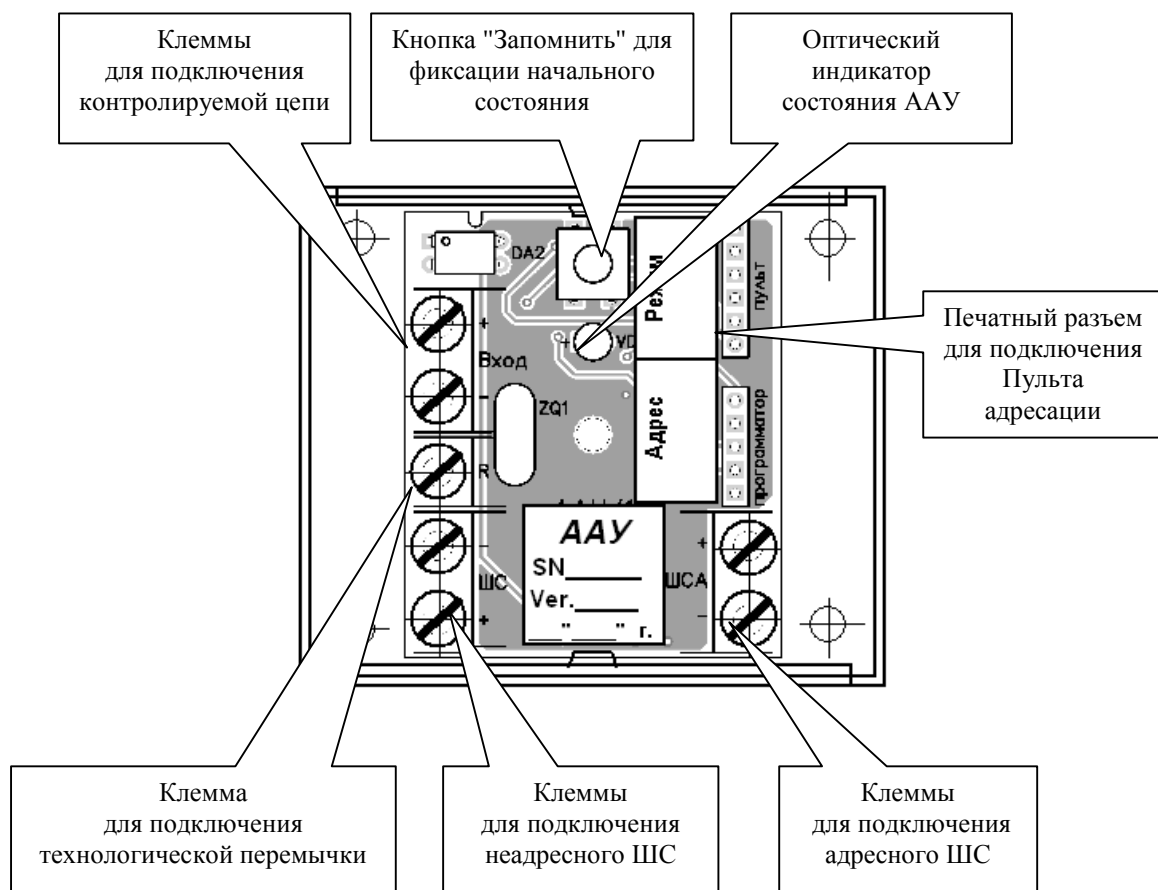
Рисунок ПЗ - Расположение и назначение клемм на плате ААУ
