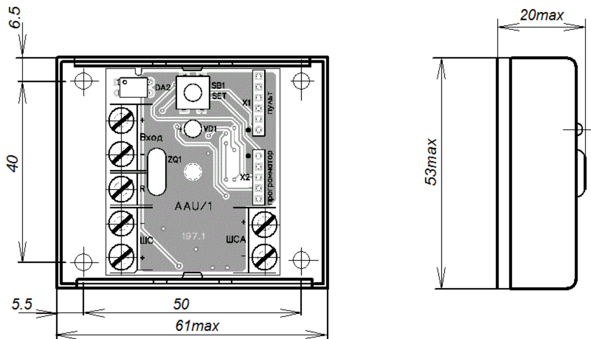
Рисунок П1 - Внешний вид, габаритные и установочные размеры ААУ
