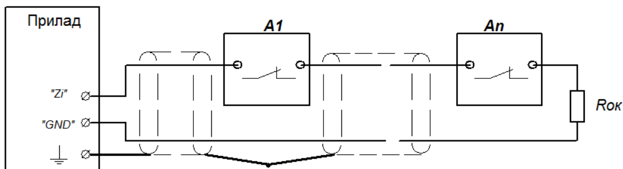
Малюнок 6.6 – Підключення НЗ охоронних пасивних сповіщувачів. Опір кінцевого резистора Rok – 5,6 кОм.
