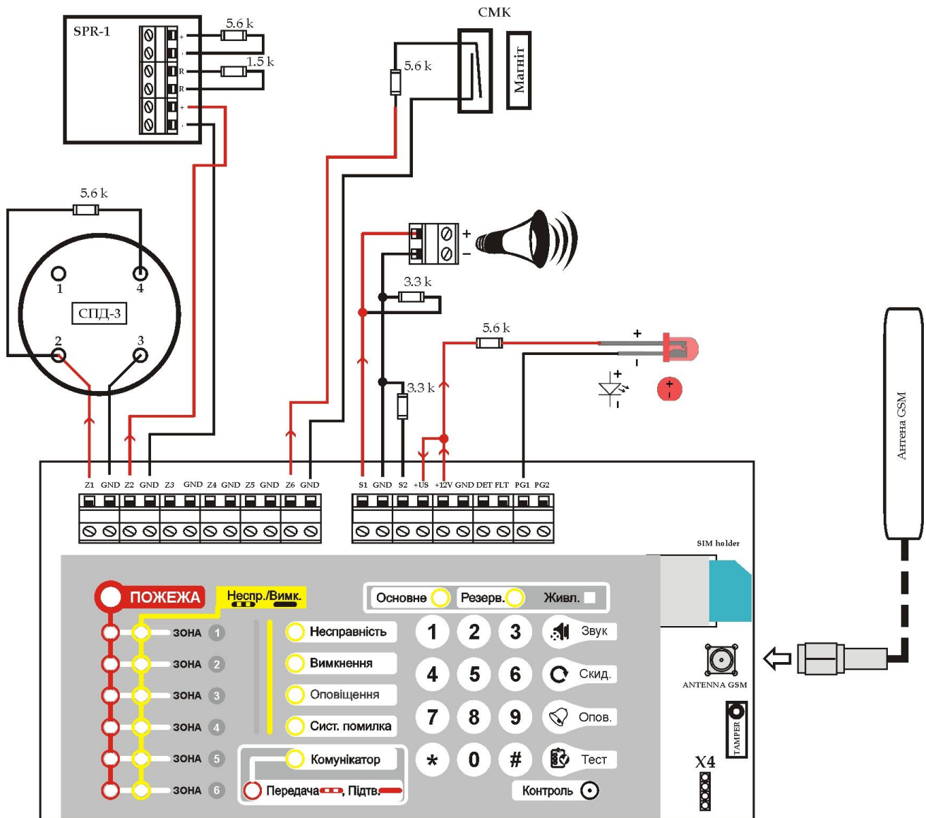
Малюнок 6.1 – Загальна схема підключення.
