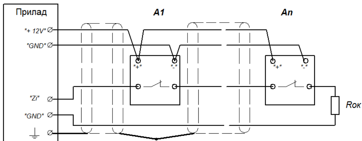
Малюнок 6.7 – Підключення НЗ охоронних активних сповіщувачів. Опір кінцевого резистора Rok – 5,6 кОм.
