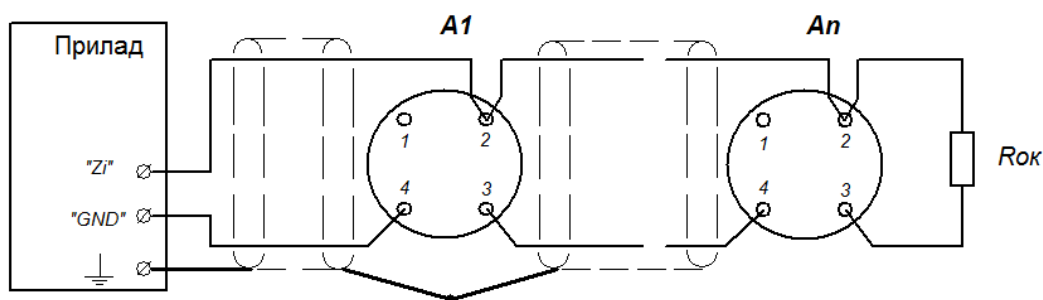
Малюнок 6.2 – Підключення димових сповіщувачів.
