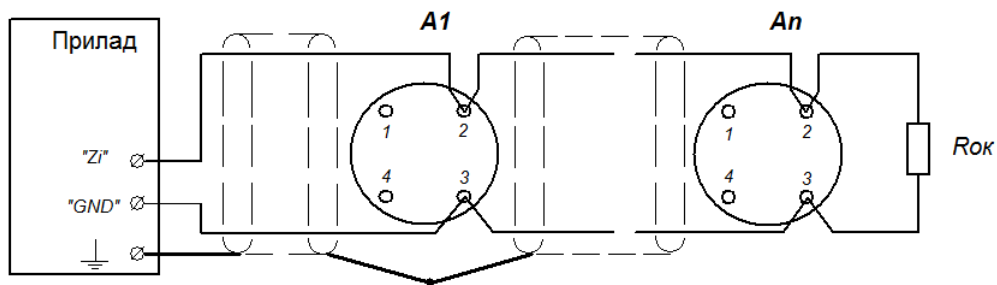
Малюнок 6.4 – Підключення теплових сповіщувачів серії FT
