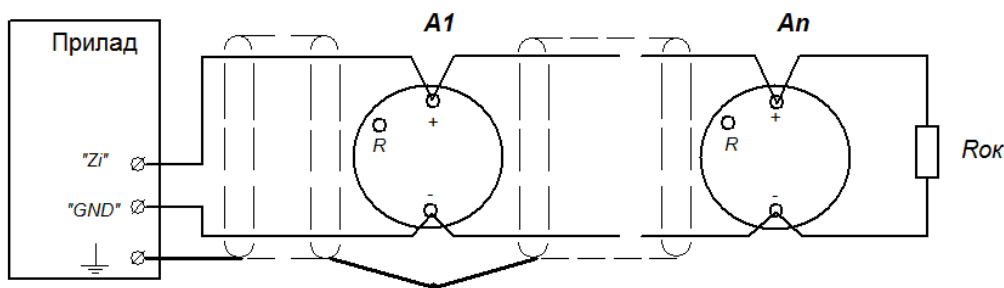
Малюнок 6.3 – Підключення теплових сповіщувачів серії ТПТ
