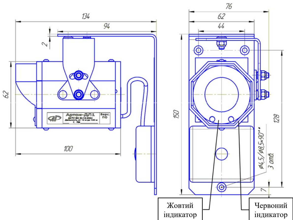
Рис.1а Блок випромінювача БВ
