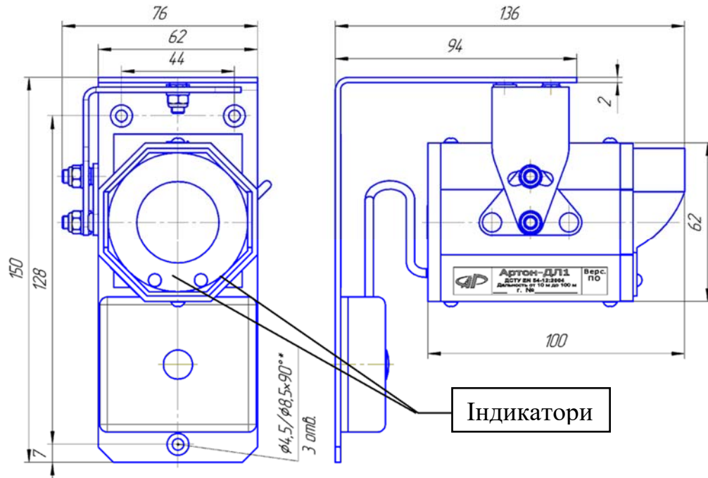
Рис.1а Блок випромінювача БВ
