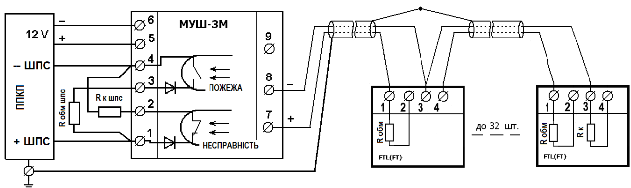
Рис. 4 Схема підключення сповіслювачів до ППКП з знакозмінним джерелом живлення ШПС
