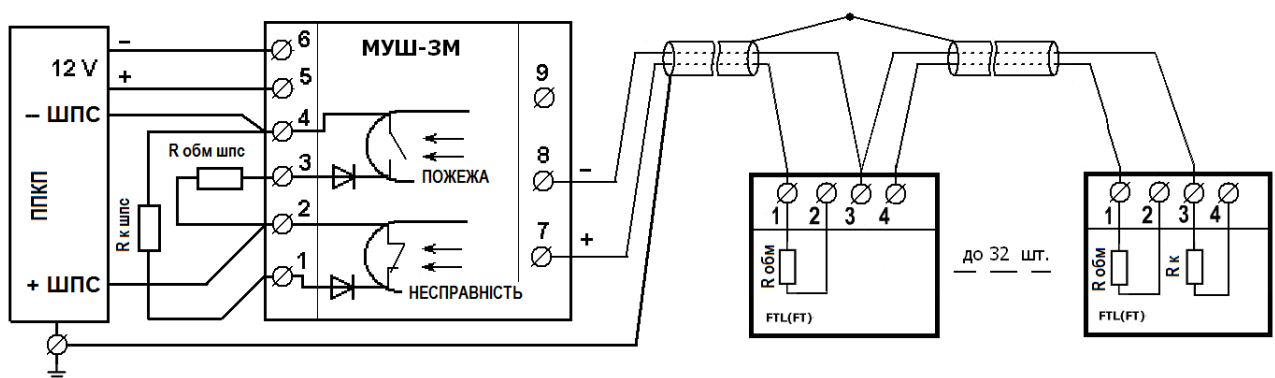
Рис. 5 Схема підключення сповіслювачів до чотирипровідного постійнострумового ШПС за допомогою модуля МУШ-3М
