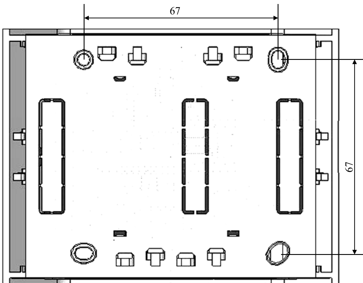
Рисунок Д7.1 – Розміщення отворів для кріплення.
