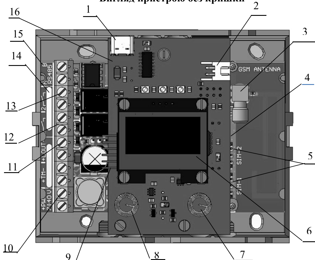
Рисунок Д2.1 - Розміщення клем та роз'ємів.
