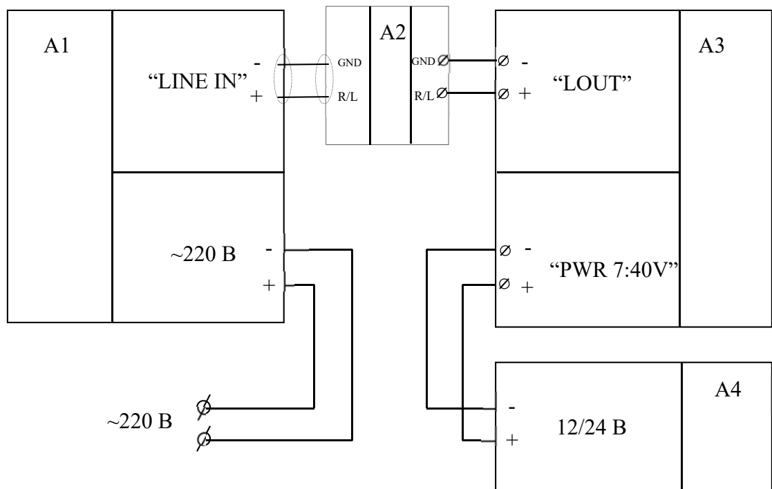
Рисунок Д5.2 – Підключення пристрою AirAlert до акустичної системи. (A1 – підсилювач, A2 – аудіо ізолятор, A3 – AirAlert, A4 – блок живлення).
