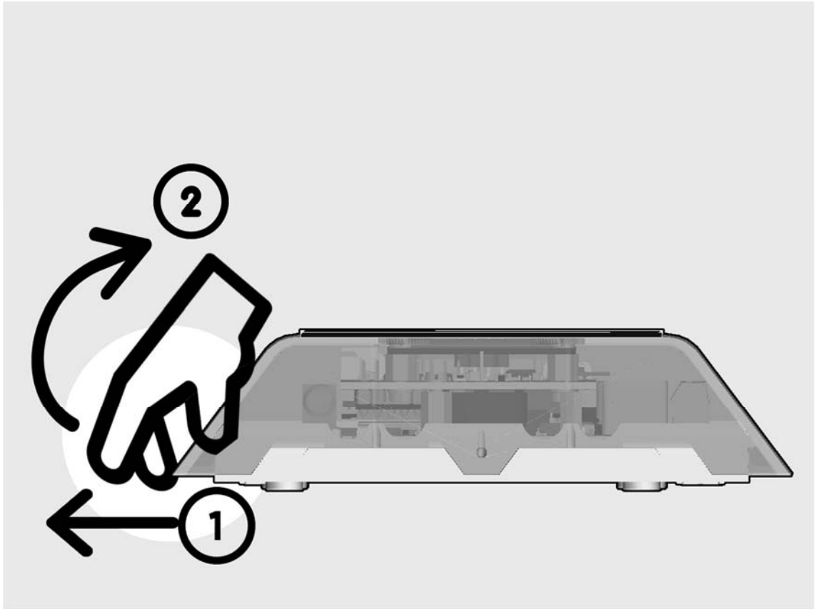
Рисунок ДЗ.1 – Зняття кришки пристрою.
