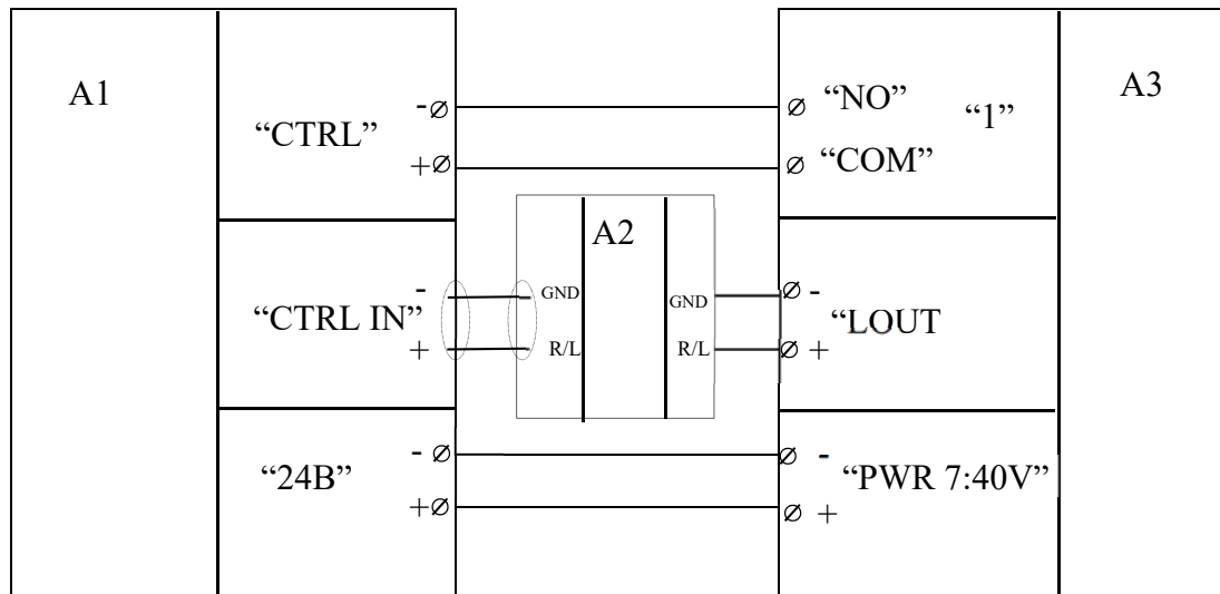
Рисунок Д5.1 – Підключення пристрою AirAlert до приладу мовленнєвого оповіщення "Vellez". (A1 – Vellez, A2 - Аудіо ізолятор, A3 – AirAlert).
