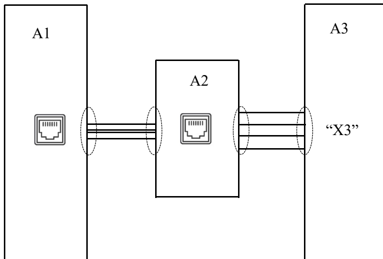
Рисунок 8 - Підключення Ethernet модуля. (A1 – Комутатор/роутер; A2 – Ethernet модуль; A3 – AirAlert;)
