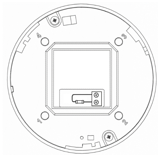
Рис 3. Встановлення обмежувального резистора
