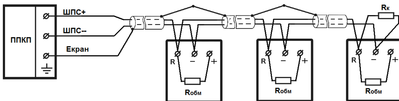
Рис. 3 Схема підключення сповіщувачів до ППКП із постійнострумовим живленням ШПС
