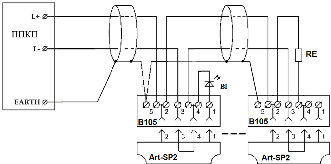
Рис. Д 7.1 – Приклад схеми підключення димових сповіщувачів типу Art-SP2 (ШС - Тип 1).
