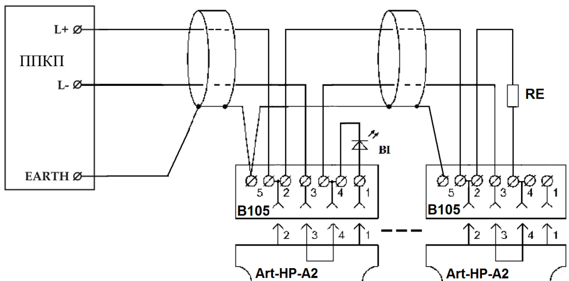
Рис. Д 7.2 – Приклад схеми підключення теплових сповіщувачів типу Art-HP-A2 (ШС - Тип 1).
