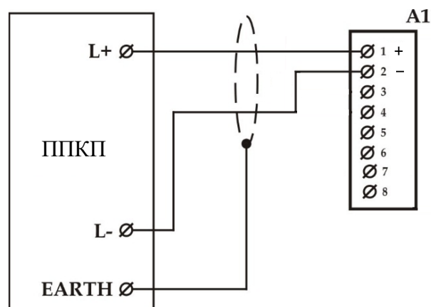
Рис. Д 7.5 – Приклад схеми підключення базової станції ArtonRL-1 (ШС - Тип 4).
