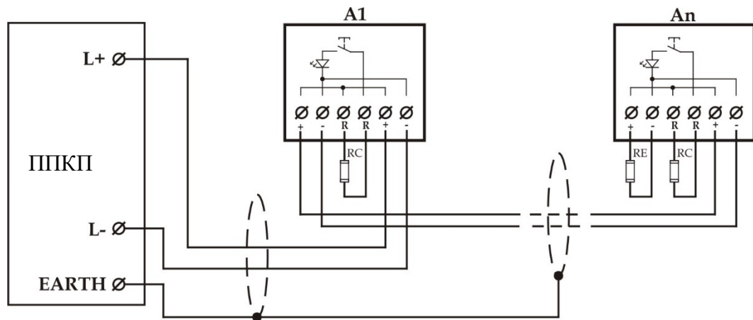
Рис. Д 7.3 – Приклад схеми підключення ручних сповіщувачів типу SPR-3LM (ШС - Тип 3).
