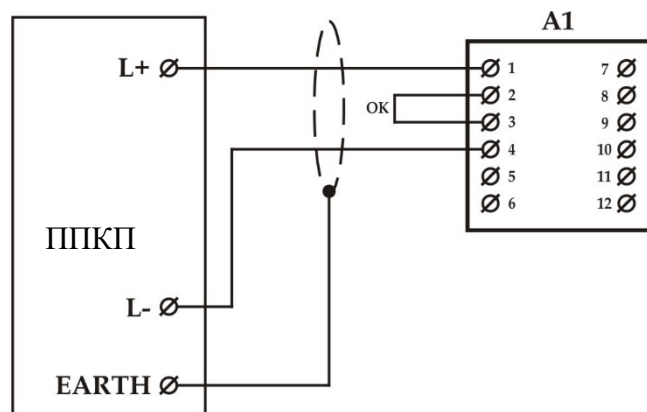
Рис. Д 7.4 – Приклад схеми підключення лінійного сповіщувача типу Art-SL3 (ШС - Тип 1 або Тип 3).
