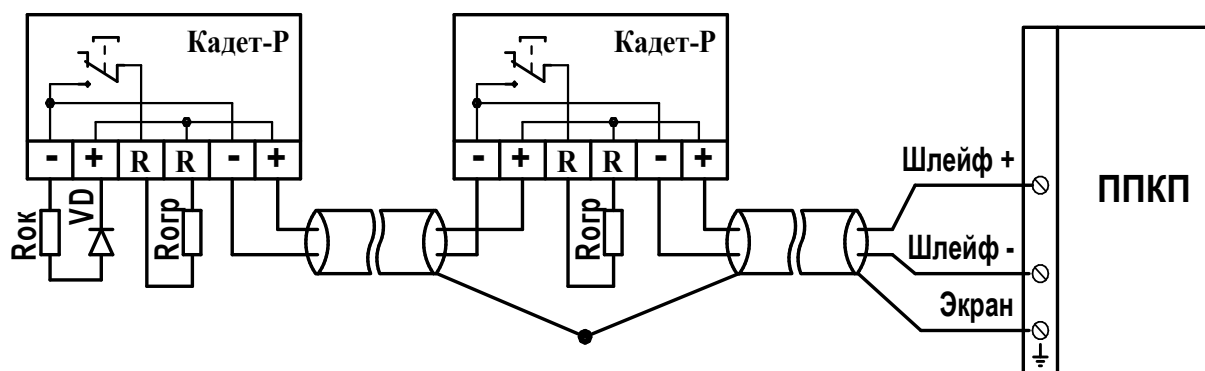
Рис. 3 Схема подключения извещателей с нормально-разомкнутым контактом к ППКП с постояннотокowym питанием ШПС (с увеличением тока в режиме «ПОЖАР»)
