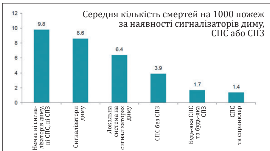
Рис. 2. Залежність кількості жертв від технічних засобів виявлення пожежі
