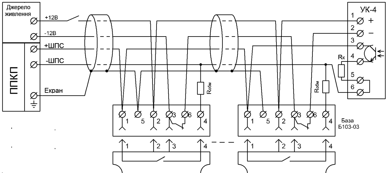
Рис. 2 Схема підключення сповісвачів до ППКП
