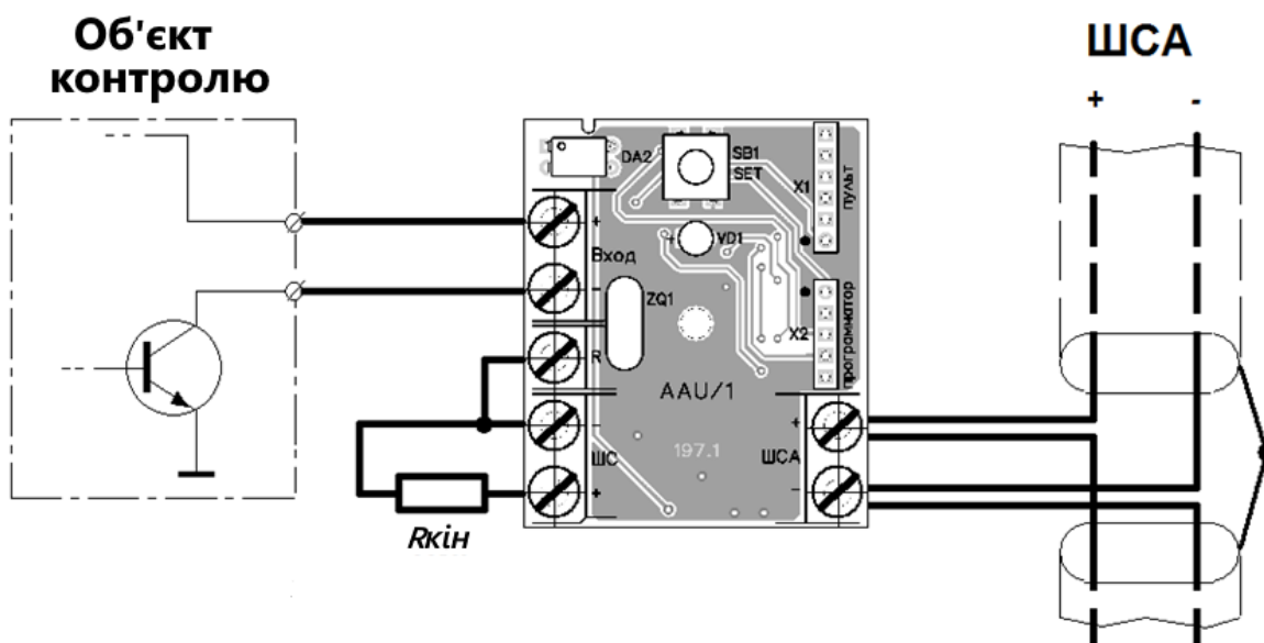
Рис. Д20.10 - Схема підключення ААУ до об'єкта контролю (сенсору) та ШСА
